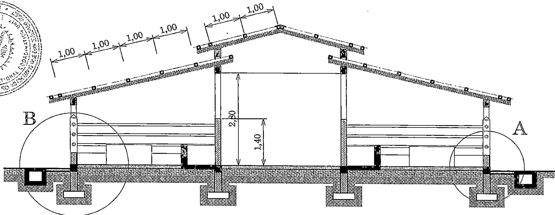
COUPE A-A
